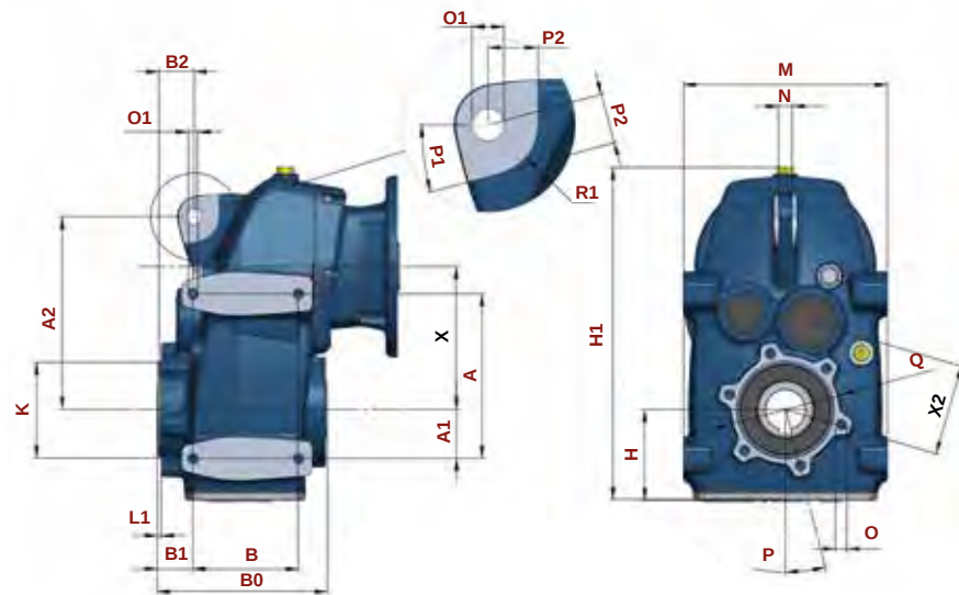
на лапах
