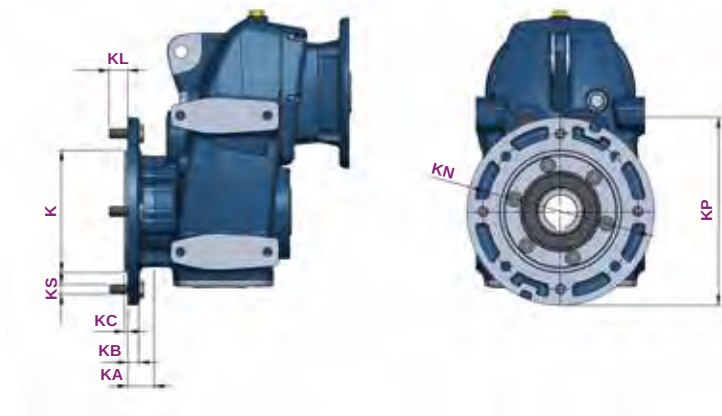
вихідний фланець
